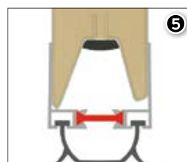
Profil bas en aluminium à rupture de pont thermique. Supprime le point de rosée.
