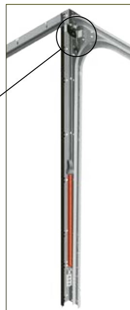
2 double-ressorts de traction intégrés dans les rails verticaux
