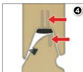
Panneaux à rupture de pont thermique composés de 2 tôles d'acier (1 int. et 1 ext.) sans point de contact.
