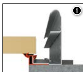
Joints latéraux et de linteau EPDM à rupture de pont thermique doublés de joints de compression.
