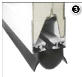
Joint bas d'étanchéité double-lèvres
